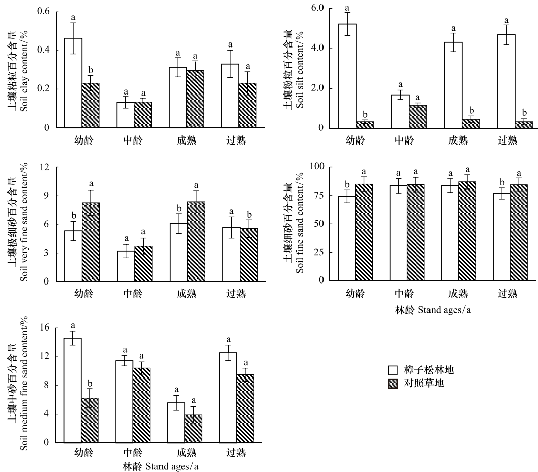
图2 樟子松林地及对照草地土壤颗粒组成差异
