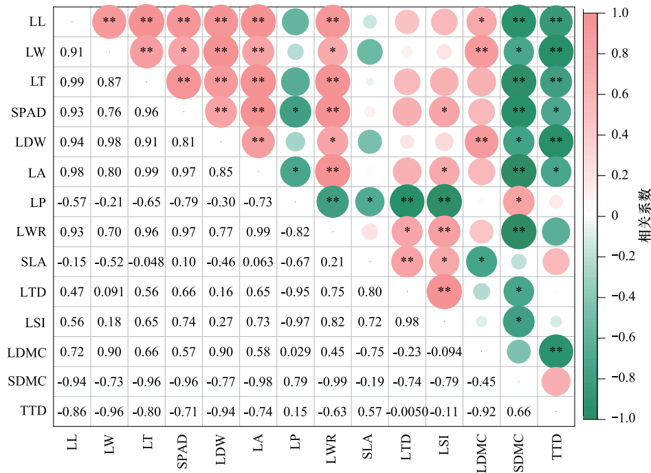
图3 14个植物功能性状指标的 Pearson 相关性热图
