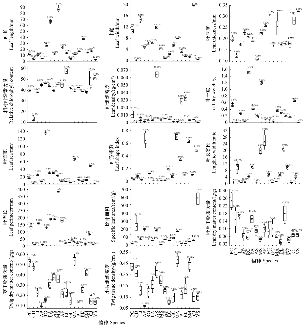
图2 长江下游 17 种滩涂湿地植物功能性状的箱线图
