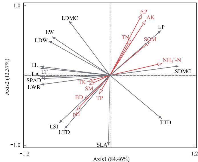
图 4 长江下游滩涂湿地优势植物功能性状与土壤因子的冗余分析(RDA)排序
