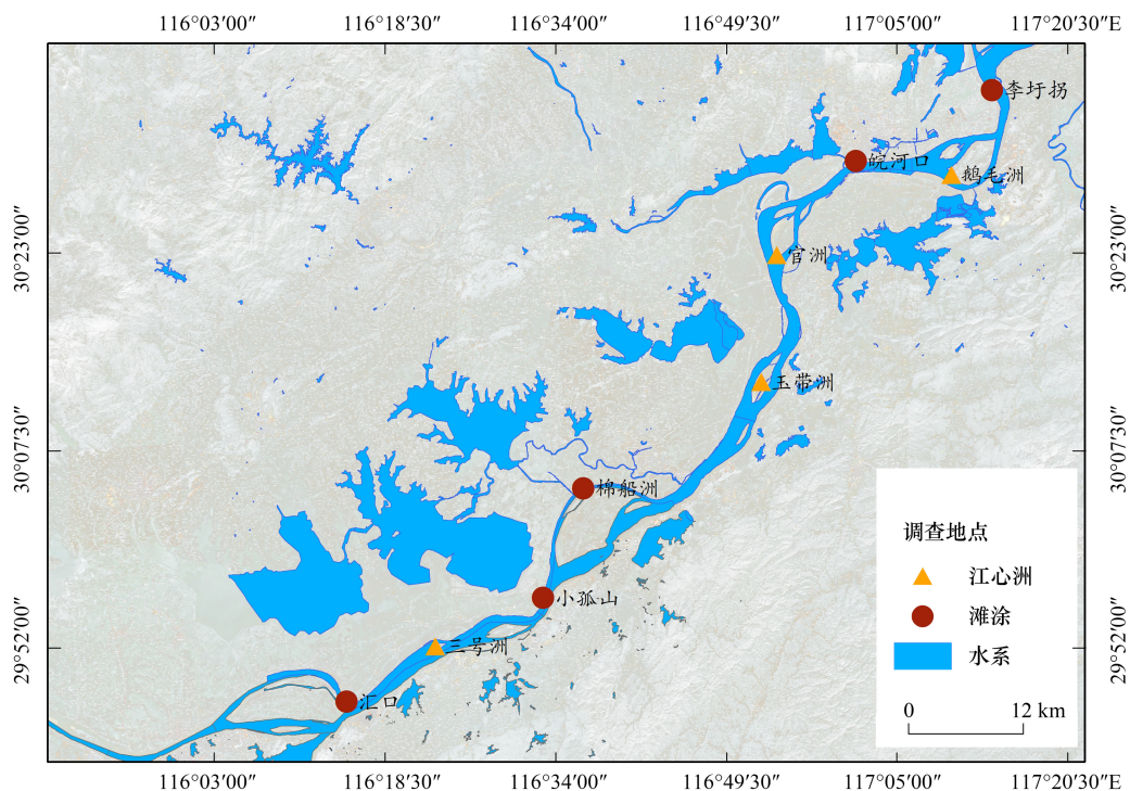
图 1 研究区分布图与采样点信息
