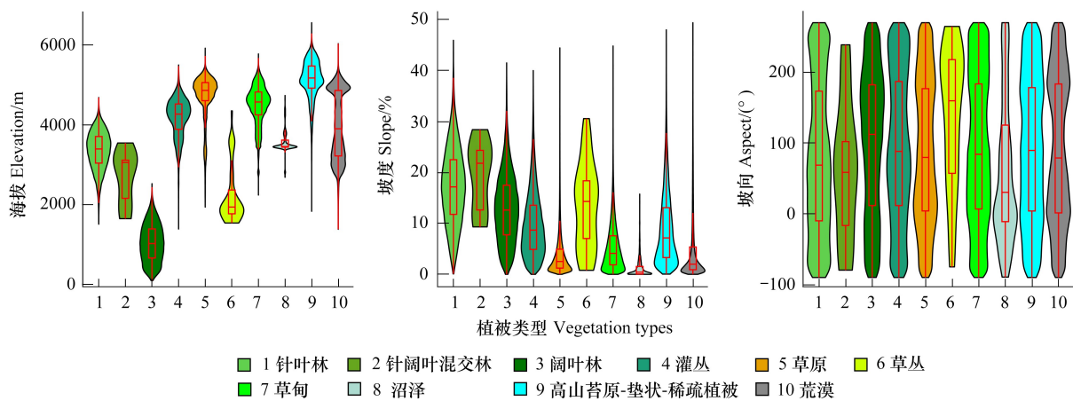
图6 不同植被类型的地形特征统计结果
