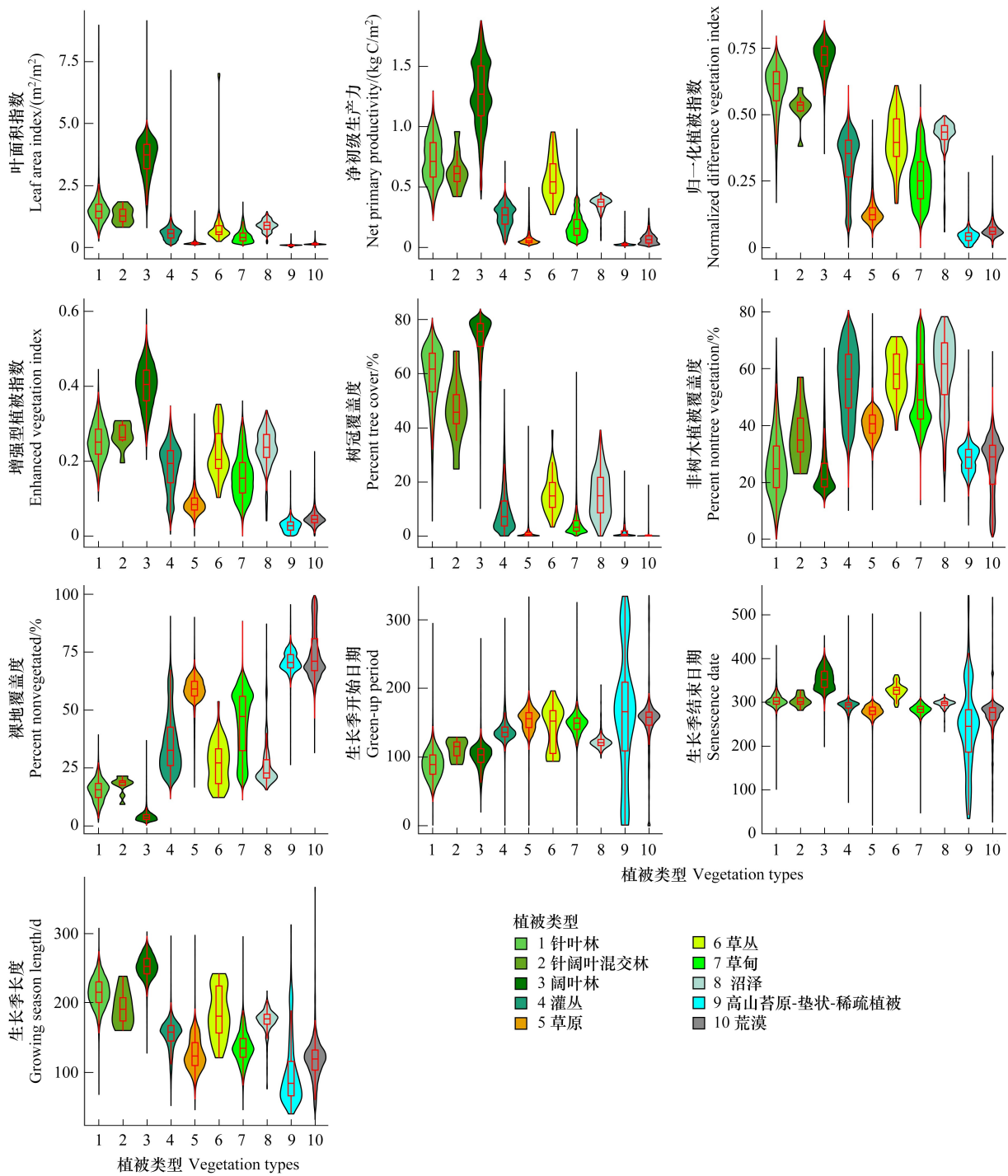
图 5 不同植被类型的植被特征统计结果
