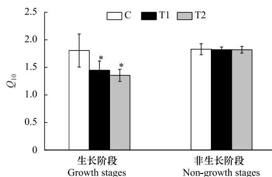
图 4 不同处理下生长阶段和非生长阶段 Q_{10} 值
