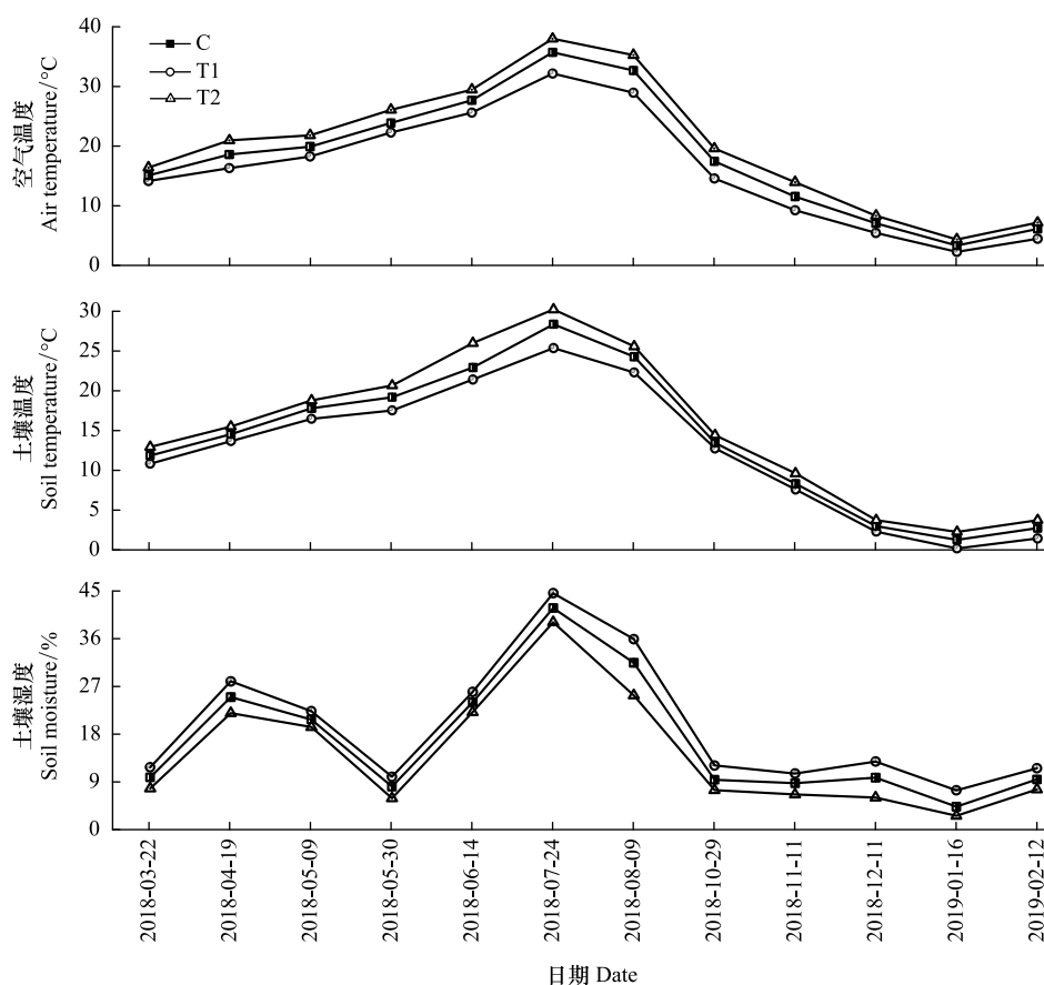
图 2 不同处理下地表空气温度、0—10 cm 土壤温度和 0—10 cm 土壤湿度
