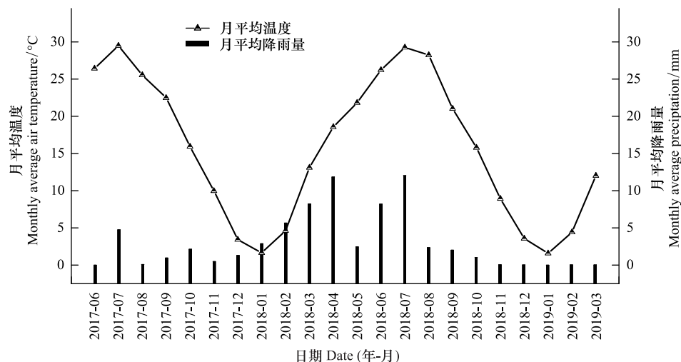
图 1 试验点的月平均大气温度和降水量变化
