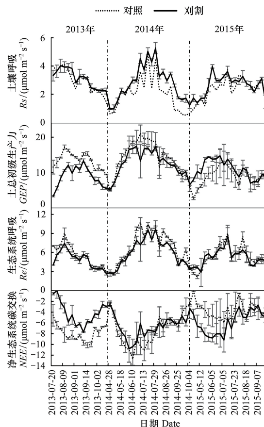
图 3 2013 年 7 月至 2015 年 10 月间生态系统 CO 2 通量各组分 的季节性变化
