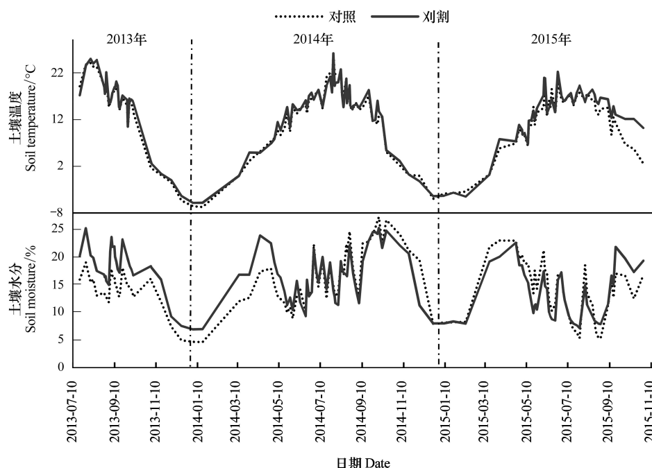
图 2 2013 年 7 月至 2015 年 10 月间 0—10 cm 日均土壤温度及水分的季节性变化
