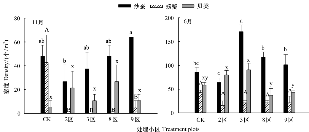
图3 2017年11月和2018年6月的大型底栖动物种类及密度
