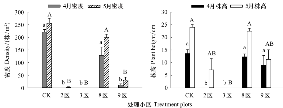
图2 互花米草克隆苗密度与株高
