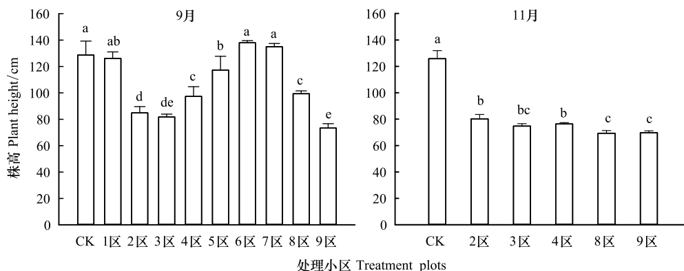
图 1 2017 年 9 月和 11 月互花米草株高
