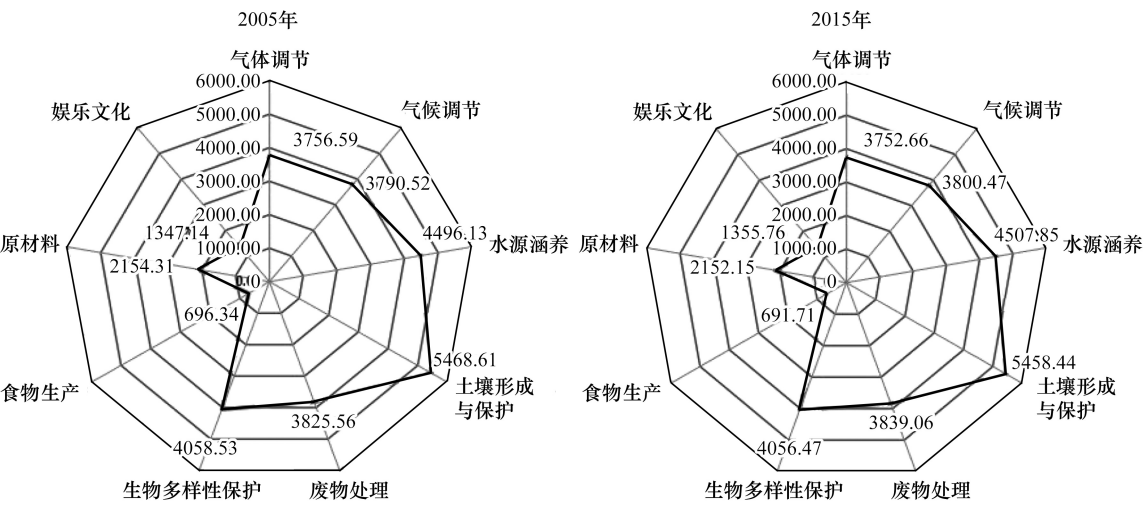
图 2 2005 和 2015 年单项 ESV/亿元雷达图 Fig.2 The radar map of single ESV/billion RMB in 2005 and 2015
