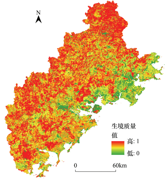
图 4 闽三角生境质量水平
