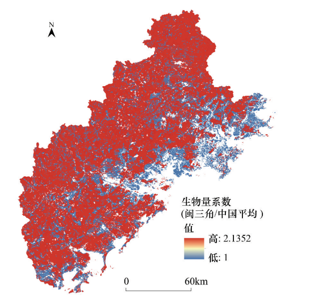
图 2 闽三角生物量系数
