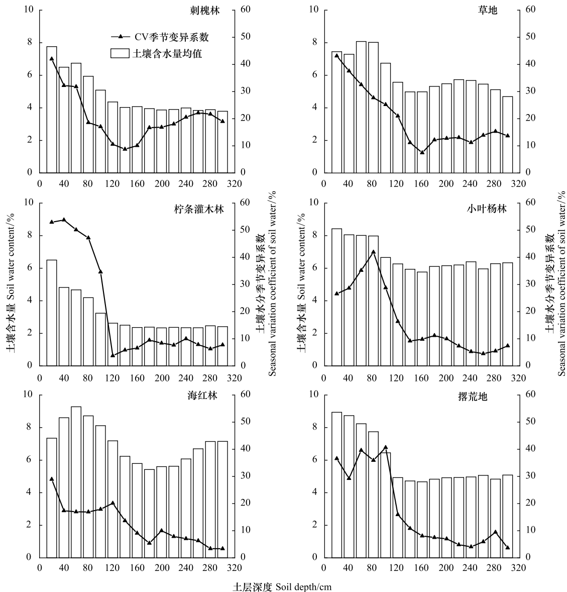
图 4 不同土地利用方式下不同土壤深度的土壤水分季节变异程度
