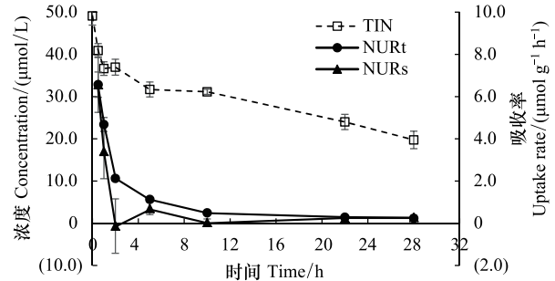
图7 海带藻片对 TIN 吸收速率的时间变化
