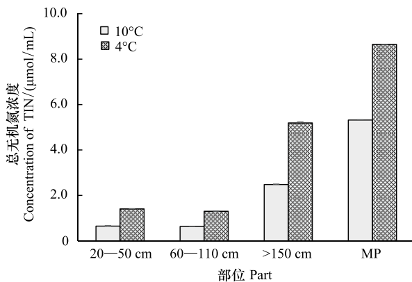
图 4 不同部位海带藻片在不同温度培养介质中 DIN 浓度的变化
