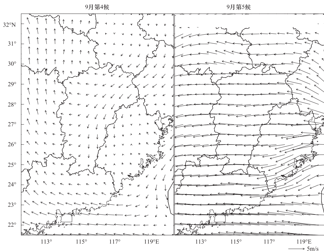
图3 2008年9月第4候与第5候平均风场分布
