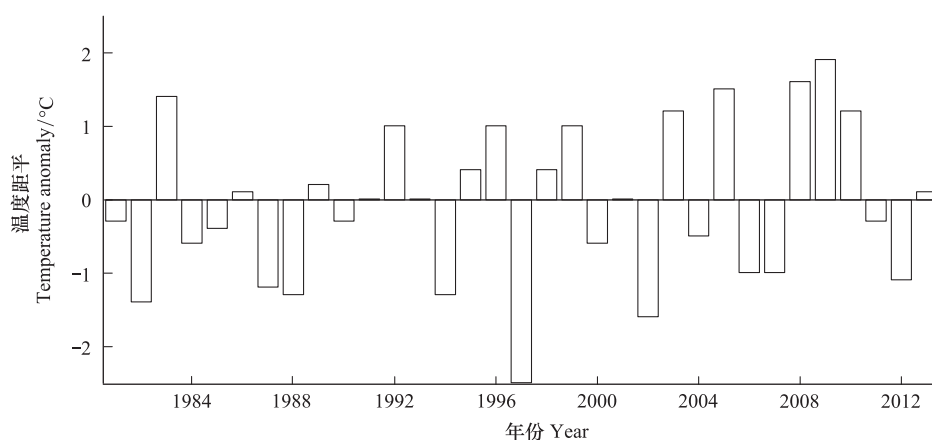
图6 1981年至2013年泰和县9月份地面温度距平
