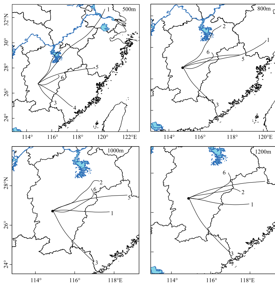
图5 2008年9月21日至9月26日泰和县回推轨迹分布
