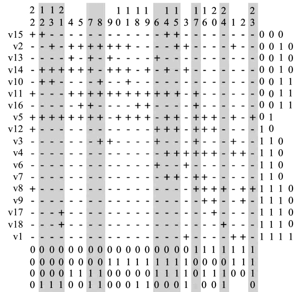
图 4 东拉山短丝木犀植物群落 TWINSpan 分类结果矩阵图
