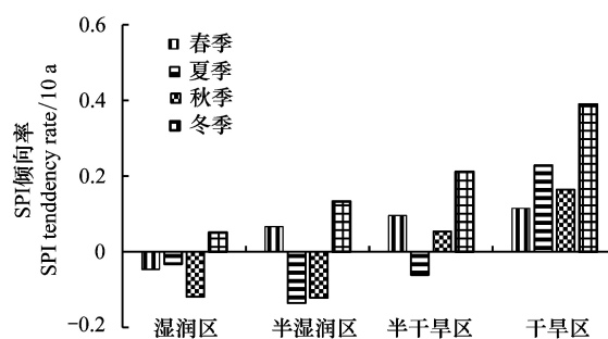
图 8 1960—2014 年不同干湿区四季 SPI 倾向率
