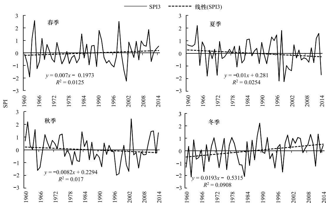
图 4 1960—2014 年北方地区四季 SPI 变化
