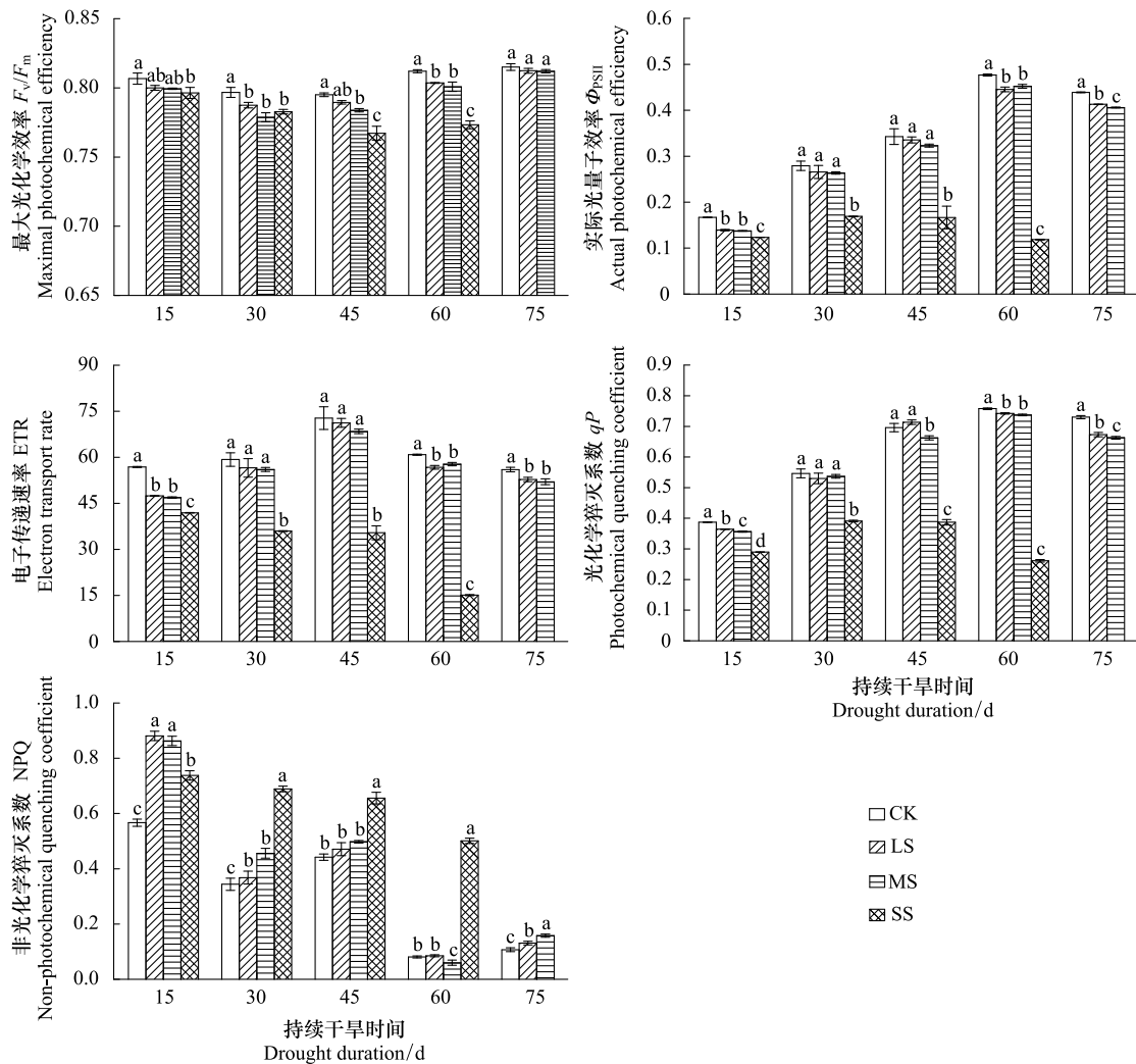
图3 不同水分处理下日本荚蒾幼苗 F_v/F_m (A)、 \Phi_{psu} (B)、ETR (C)、 qP (D)、NPQ (E) 的变化
