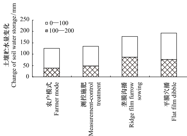
图5 不同覆膜方式下冬小麦种植前后0—100cm与100—200cm土层土壤水分的消耗情况
