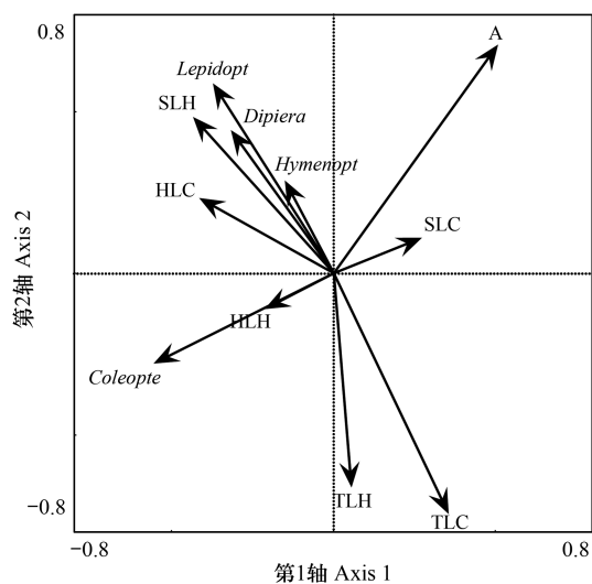
图 5 传粉昆虫-环境因子 RDA 排序图
