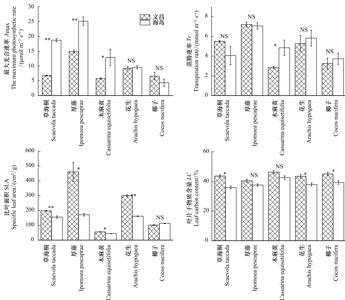
图 1 5 种植物在热带珊瑚岛和文昌的最大光合速率 A_{\max} (a), 蒸腾速率 T_r (b), 比叶面积 SLA (c), 叶片碳含量 LC (d) (平均值 \pm 标准误差)
