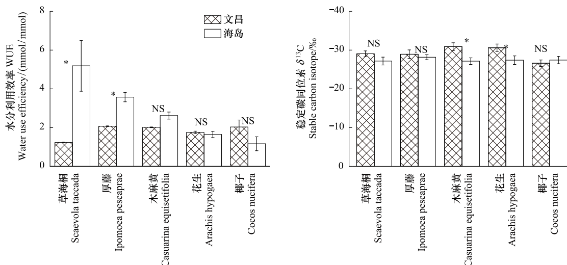
图 2 5 种植物在热带珊瑚岛和文昌的瞬时水分利用效率 WUE (a), 稳定碳同位素含量 \delta^{13}\text{C} (b) (平均值 \pm 标准误差)
