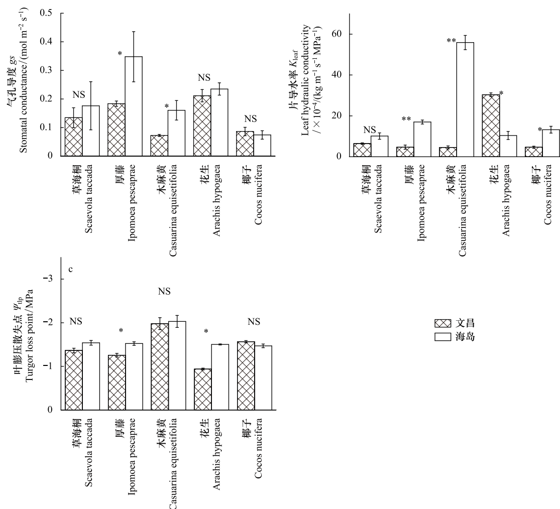
图3 5种植物在热带珊瑚岛和文昌的气孔导度 g_s (a), 叶片导水率 K_{leaf} (b), 膨压丧失点 \Psi_{lp} (c) (平均值±标准误差)
