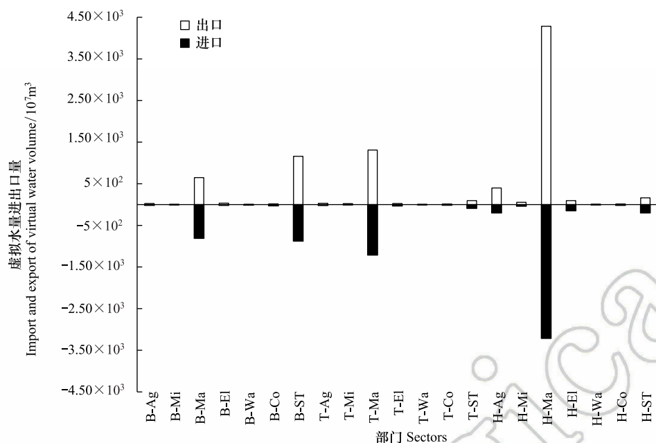
图3 京津冀各部门进虚拟水进出口量
