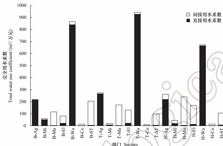
图1 京津冀各部门直接、间接及完全用水系数
