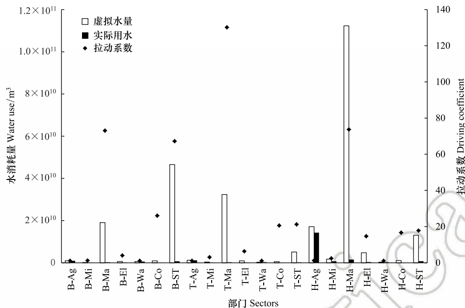
图2 京津冀各部门消耗虚拟水量、生产实际用水量及拉动系数
