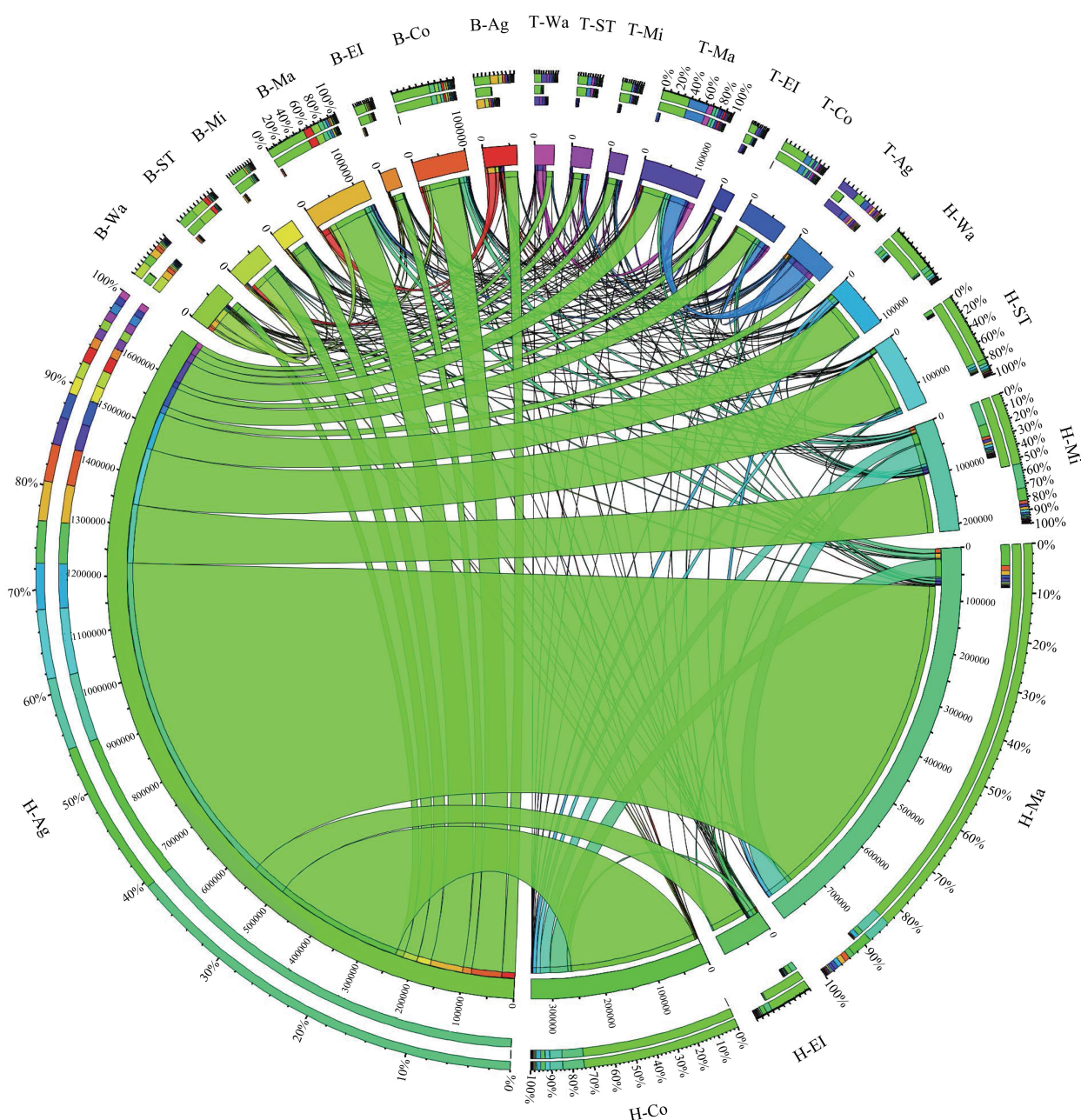
图5 京津冀各部门间虚拟水流动分布图/ 10^4 \text{ m}^3
