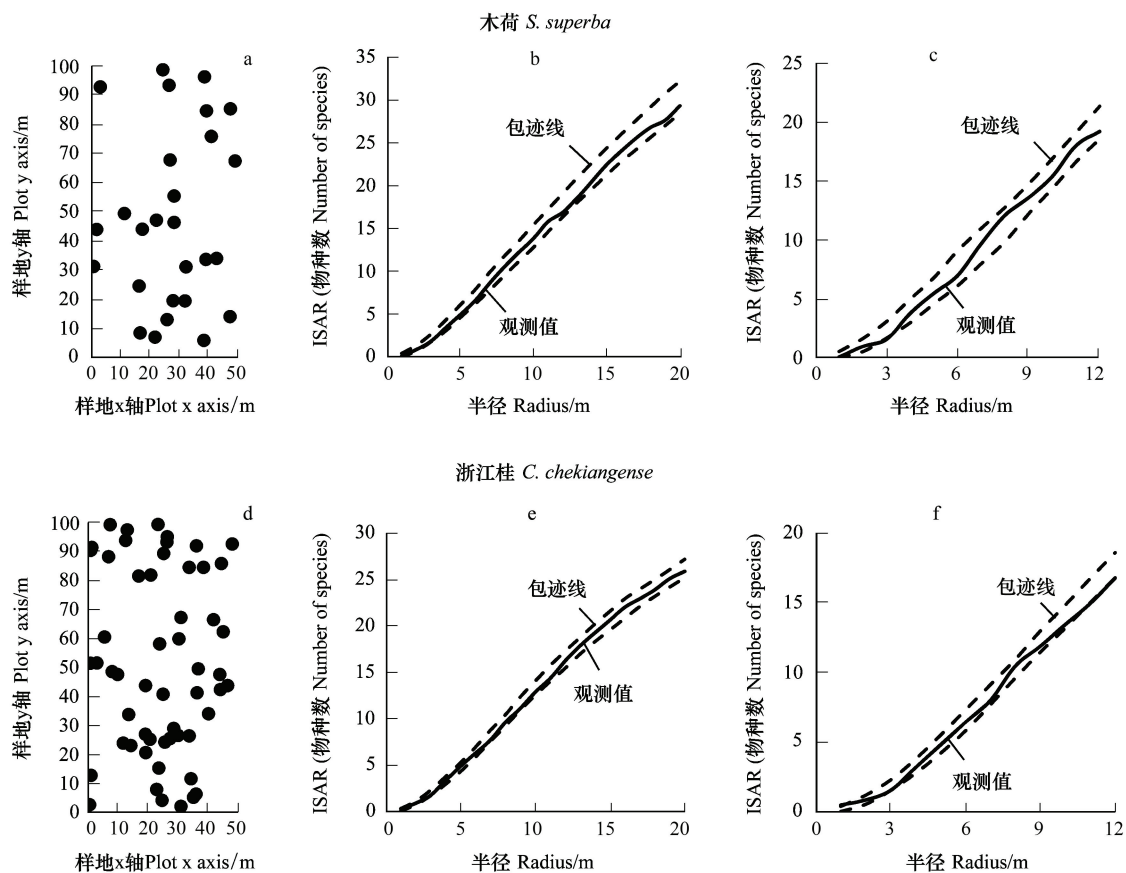
图 1 两个示例种的空间分布及其单物种-面积关系 (individual species-area relationship, ISAR) 分析
