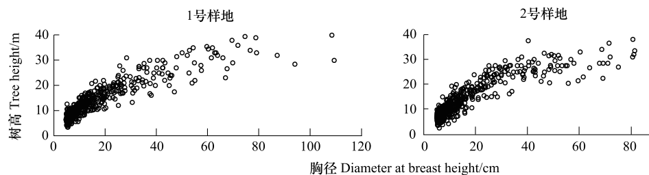
图4 样地林木树高-胸径关系散点图
