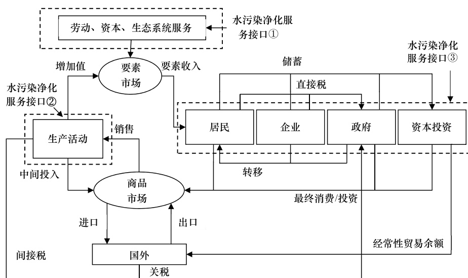
图 1 ES-CGE 模型基础框架
