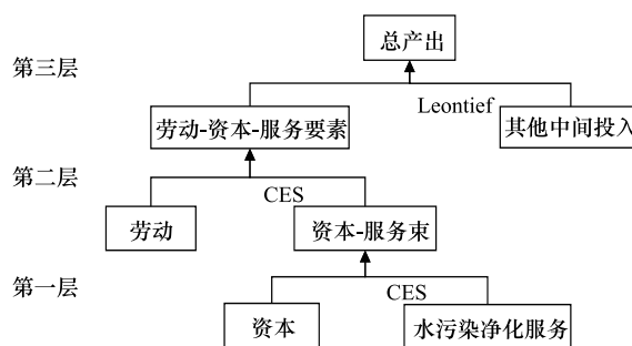
图3 劳动-资本-服务生产函数结构
