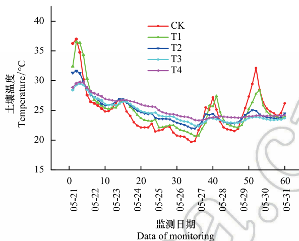
图 7 不同处理措施下表层 5cm 处土壤温度变化
