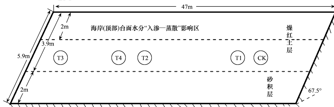
图 2 试验区原位小区布设示意图
