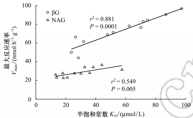
图3 土壤 \beta\text{-1,4} -葡萄糖苷酶 ( \beta\text{G} ) 和 \beta\text{-1,4-N} -乙酰葡萄糖苷酶 (NAG) 动力学参数 V_{\max} 、 K_m 的相关性分析
