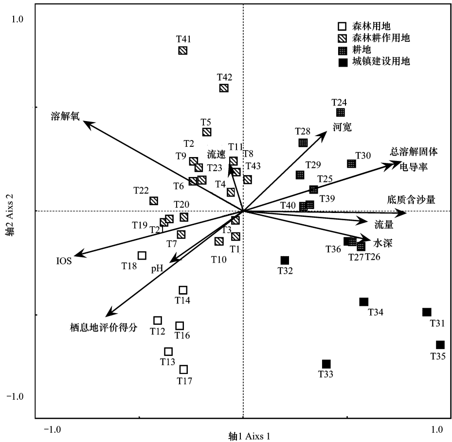
图 3 太子流域鱼类群落结构与环境因子的典范对应分析
