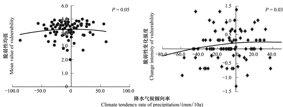
图7 年降水气候倾向率与近13年平均脆弱性值和脆弱性变化强度的相关性
