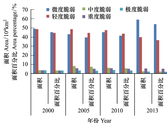
图4 西南喀斯特山区近13年不同等级脆弱性面积对比
