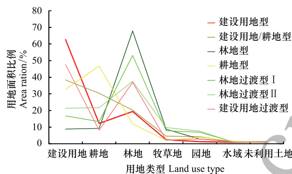
图 6 二次聚类结果的土地利用类型比例
