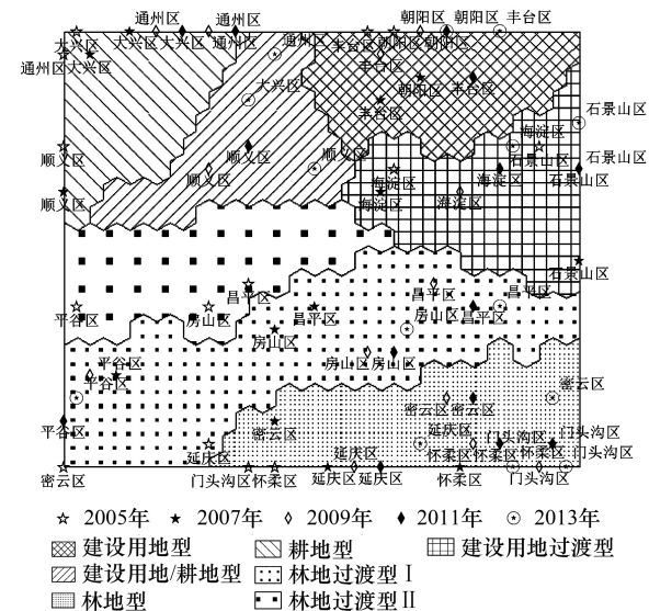
图 5 二次聚类 SOM 面板区域划分
