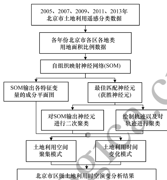
图 2 总体技术流程图
