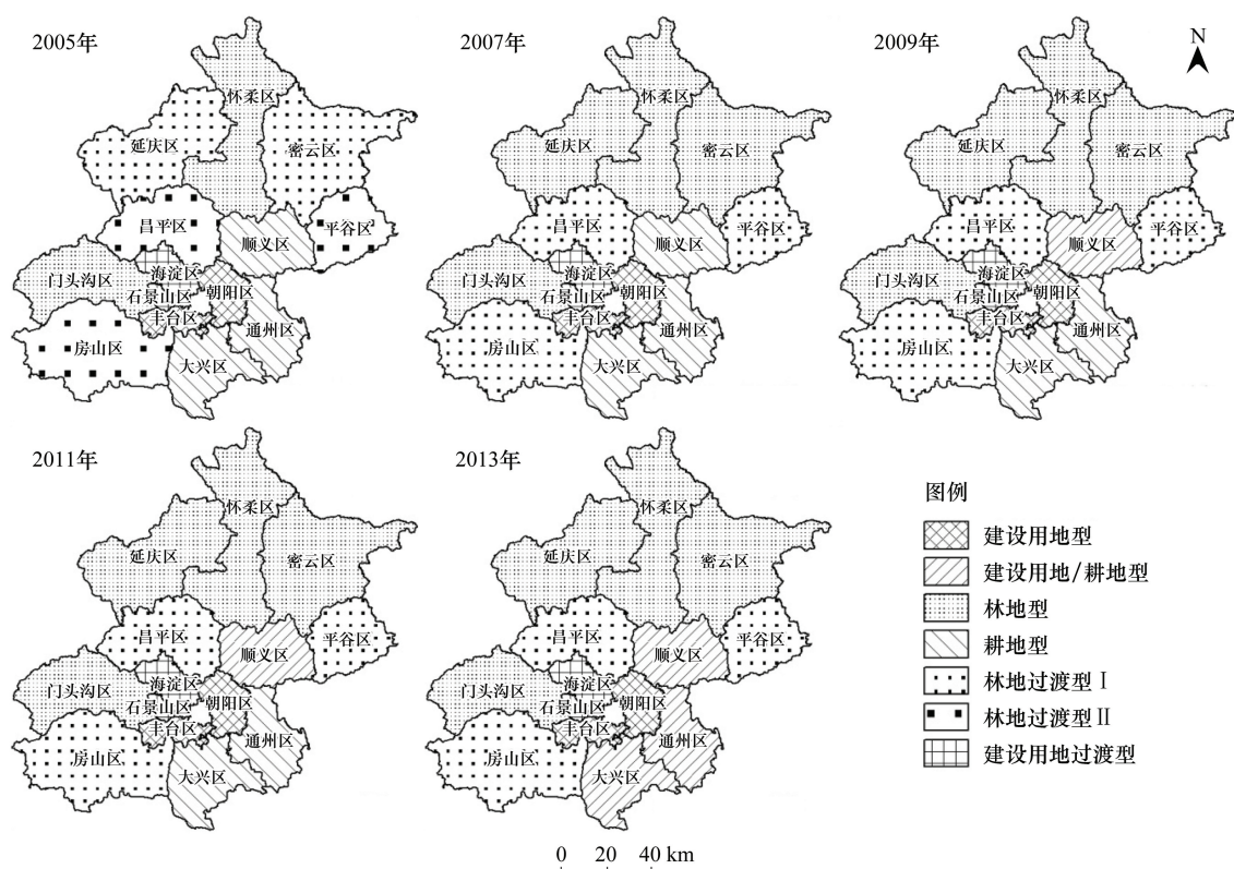
图 7 不同年份的聚类结果在地理空间中的可视化
