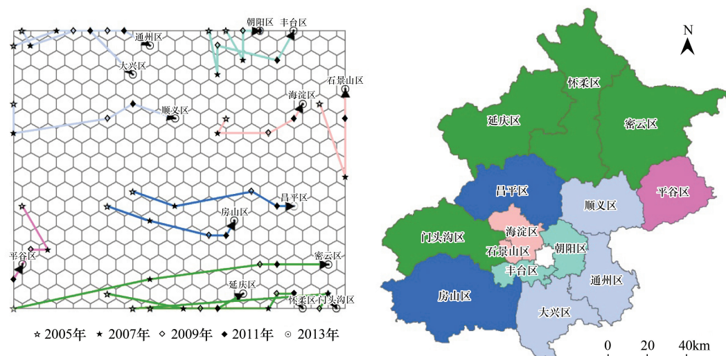
图 8 土地利用变化轨迹与可视化
