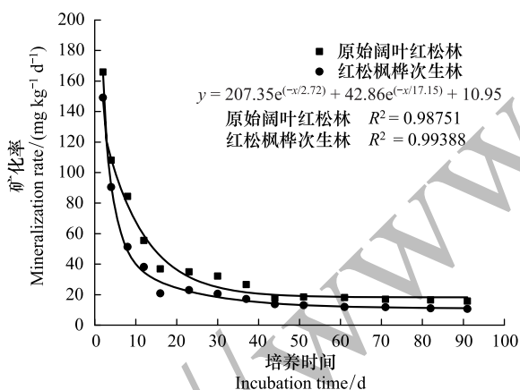
图 2 中生演替系列土壤有机碳矿化率
