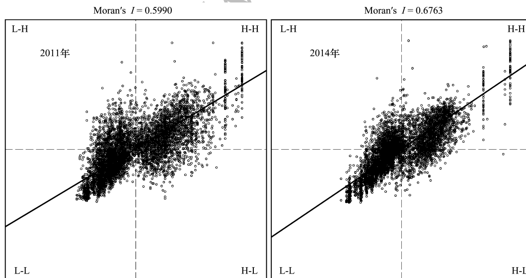
图 4 Moran 散点图
