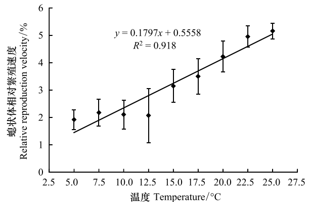
图 3 温度对海月水母螅状体相对繁殖速度的影响
