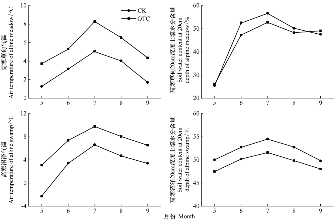
图 1 高寒草甸和沼泽草甸 OTC 内外的生长季内月平均气温及 20cm 土层含水量
