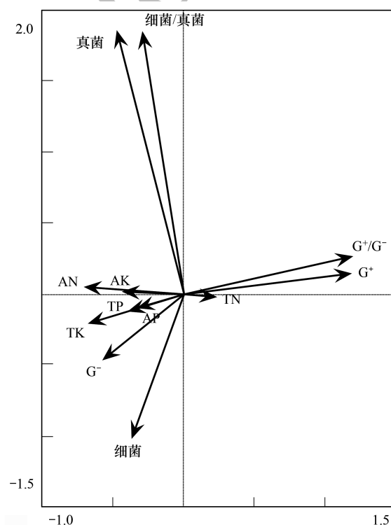
图2 不同连作年限牛膝根际土壤中各类 PLFAs 和大量元素冗余分析
