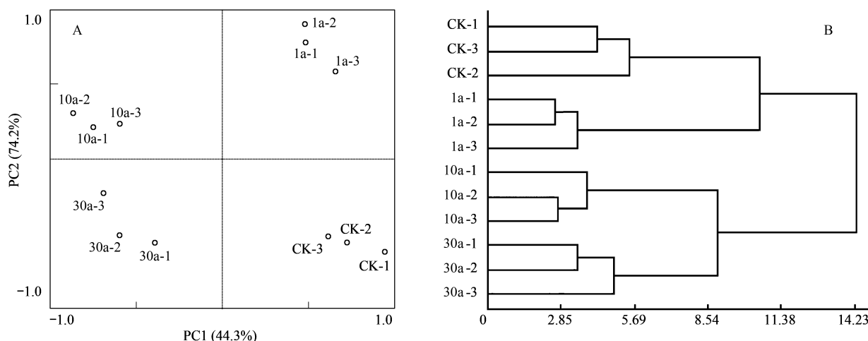
图1 不同连作年限牛膝根际土壤中 PLFAs 生物标记主成分分析(A)和聚类分析(B)
