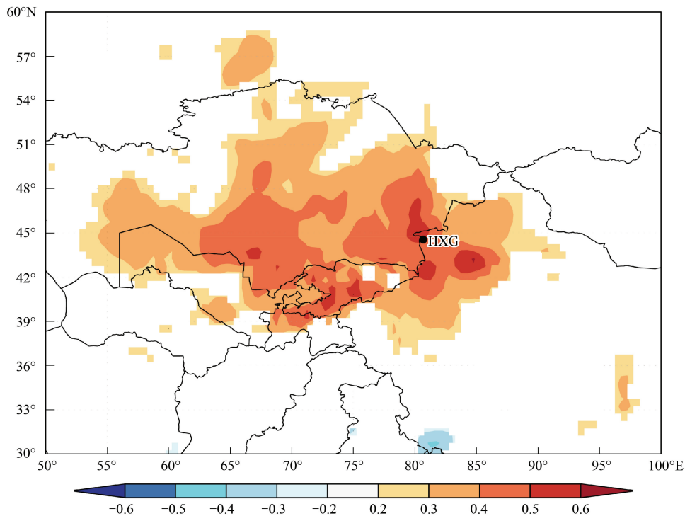
图 8 赛里木湖降水重建序列与 CRU 上年 8 月到当年 7 月降水量的空间相关 (1960—2009, P < 10\% )
