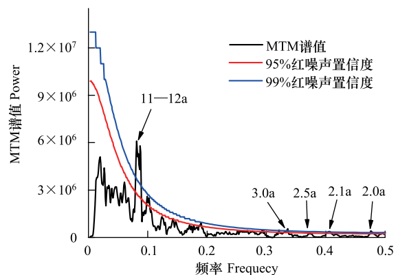
图 6 重建序列的多窗谱分析
