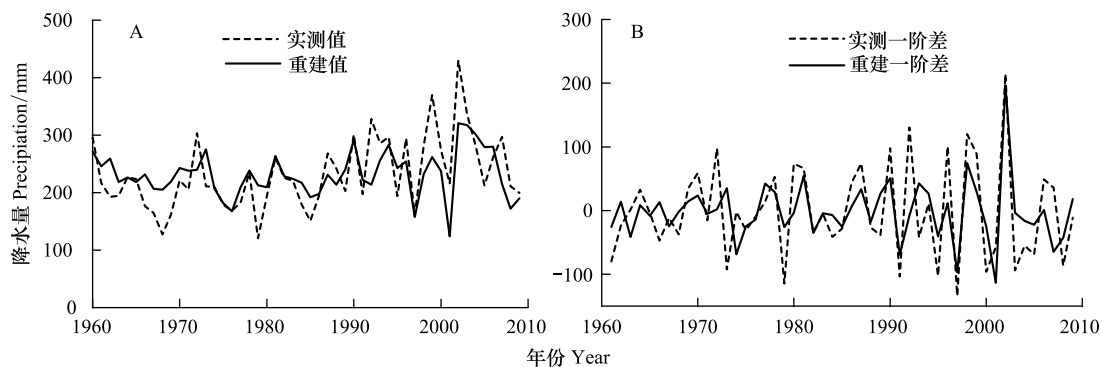
图 5 重建序列与实测序列的对比
