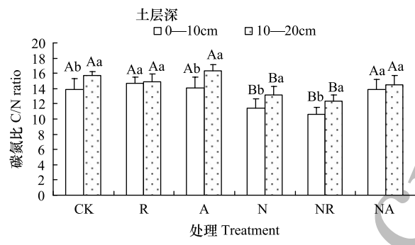
图4 模拟氮沉降和降雨对土壤碳氮比的影响
