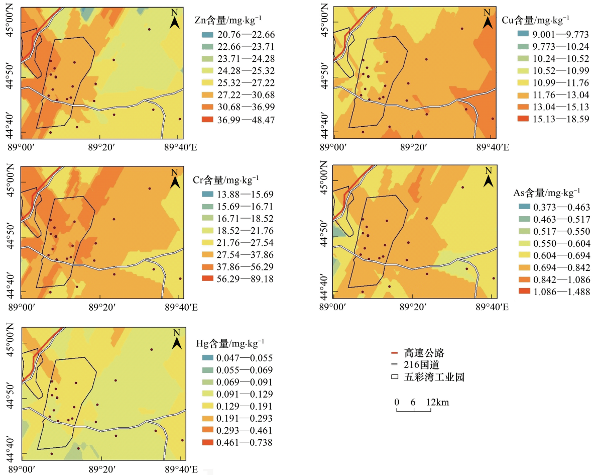
图2 琵琶柴重金属空间分布图
