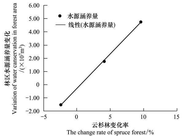
图 7 云杉林变化率与林区水源涵养关系图
