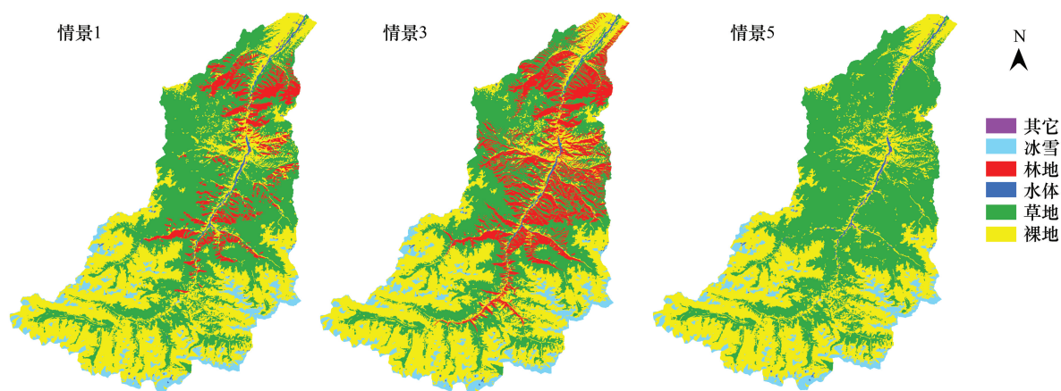
图 3 不同情景土地利用类型图
