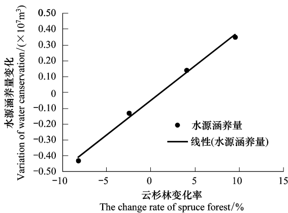
图 6 云杉林变化率与研究区水源涵养关系图
