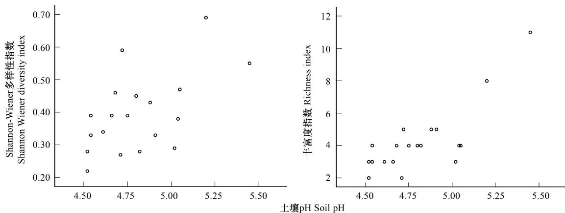
图 4 物种 Shannon-Wiener 多样性指数 H' (左) 及物种丰富度指数 S (右) 与土壤 pH 值关系
