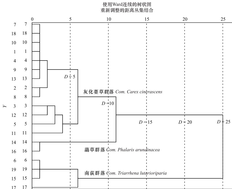
图 2 恒湖农场茶叶港草洲 19 个样地聚类分析树状图
