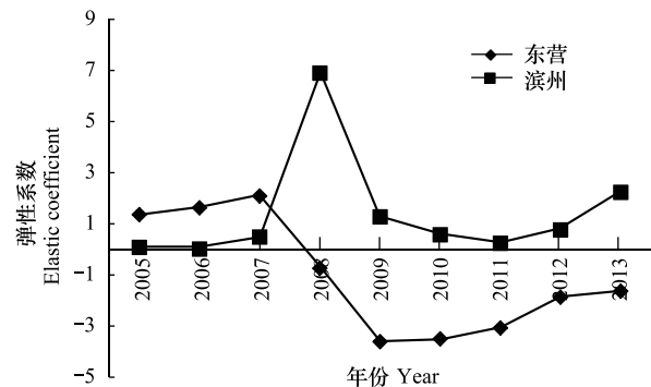
图 5 东营和滨州碳排放生态足迹主要抑制因素变化
