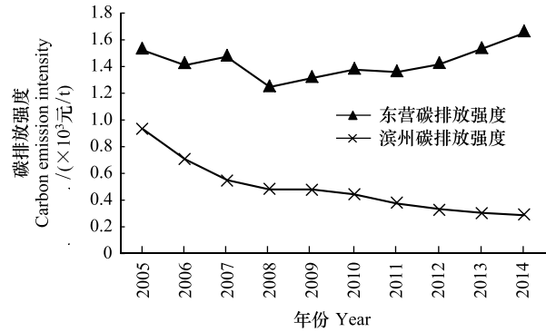
图 3 东营和滨州碳排放强度变化图
