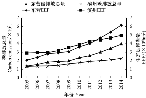
图 2 东营和滨州碳排放和生态足迹变化图
