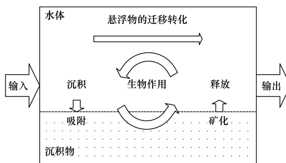
图1 河流内部磷素迁移转化的主要过程
