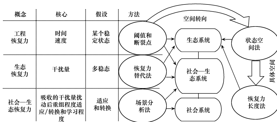
图5 恢复力理论及测量方法演变
