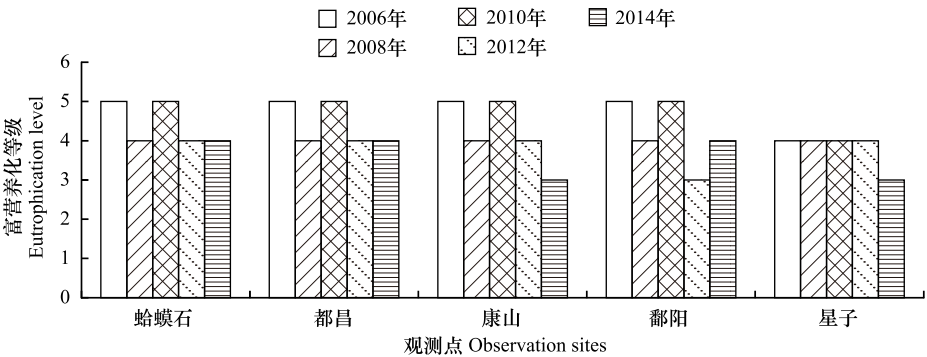
图 1 鄱阳湖流域 5 个主要观测点 5 年水体富营养化等级变化趋势
