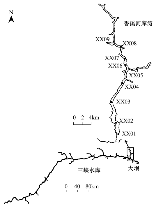
图 1 三峡水库香溪河库湾样点设置
