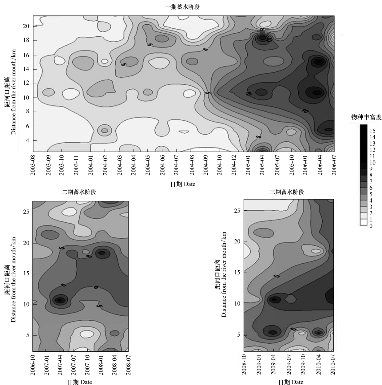
图3 三个蓄水阶段香溪河库湾平均底栖动物物种丰富度的变化对比 (a:一期蓄水阶段;b:二期蓄水阶段;c:三期蓄水阶段)
