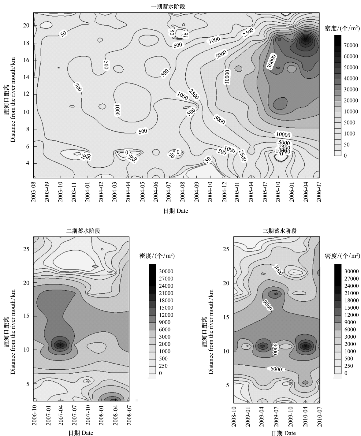
图 2 三个蓄水阶段库湾平均底栖动物密度的变化对比 (a: 一期蓄水阶段; b: 二期蓄水阶段; c: 三期蓄水阶段)
