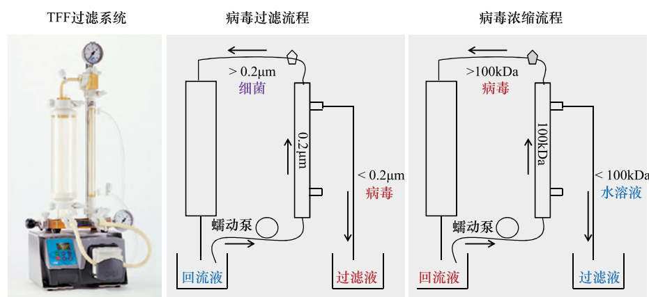
图 2 TFF 过滤系统及流程 [13]
