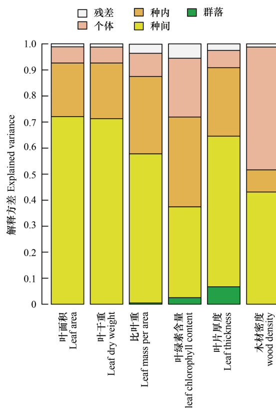
图 2 功能性状的在个体、种内、种间及群落水平的方差分解
