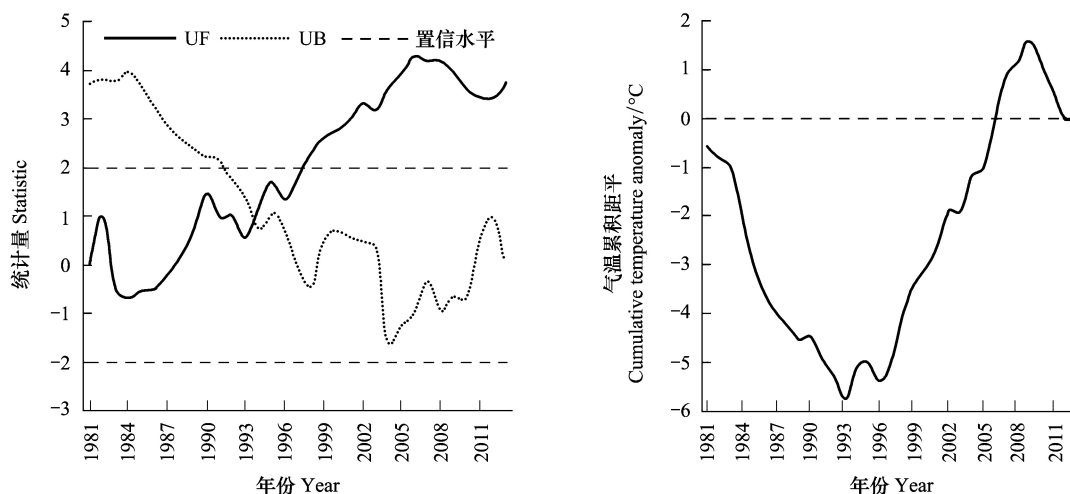
图 6 年均温 M-K 检测与累积距平图
