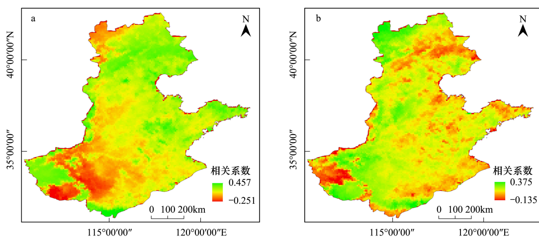
图 14 植被覆盖度与当月温度 (a) 和降水量 (b) 的相关系数
