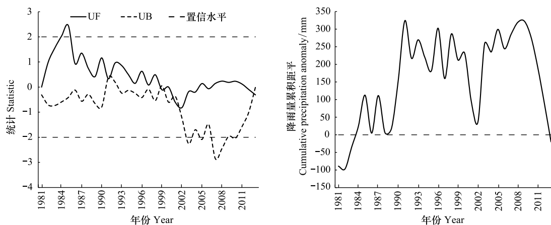
图7 年均降水量 M-K 检测与累积距平图
