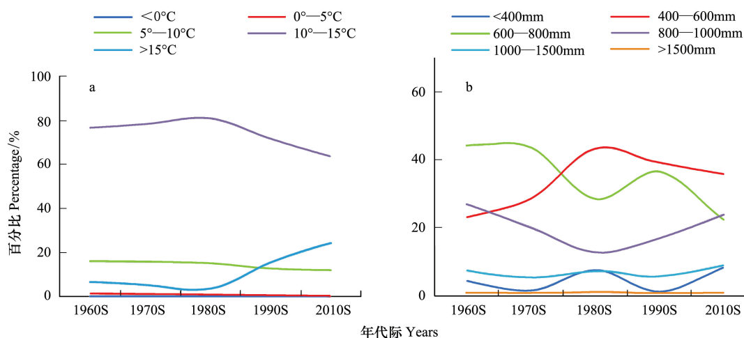
图 5 华北平原气温 (a) 与降水量 (b) 各统计量变化趋势图
