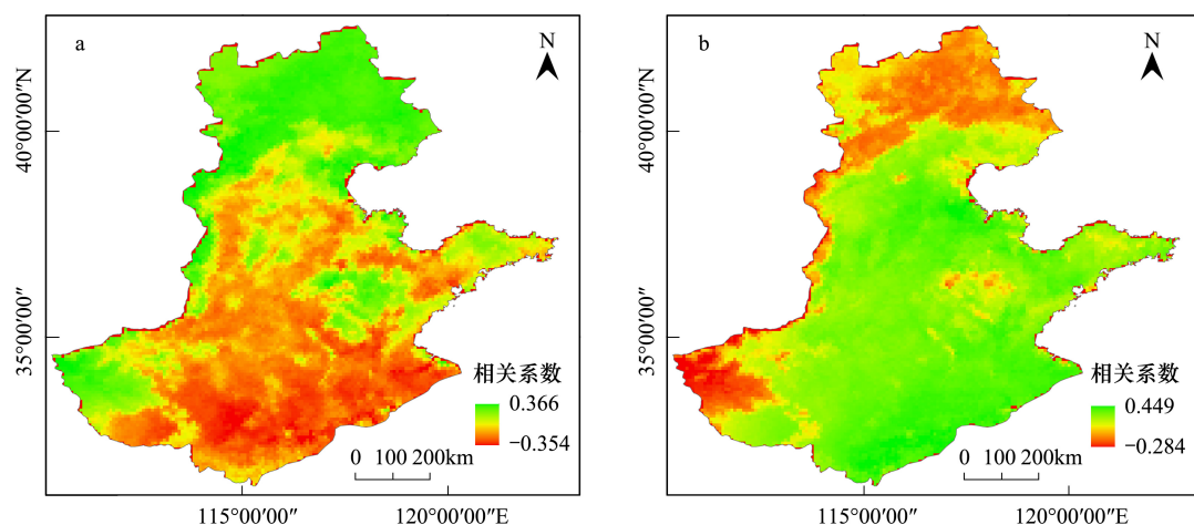
图 15 植被覆盖度与前一月温度 (a) 和降水量 (b) 的相关系数
