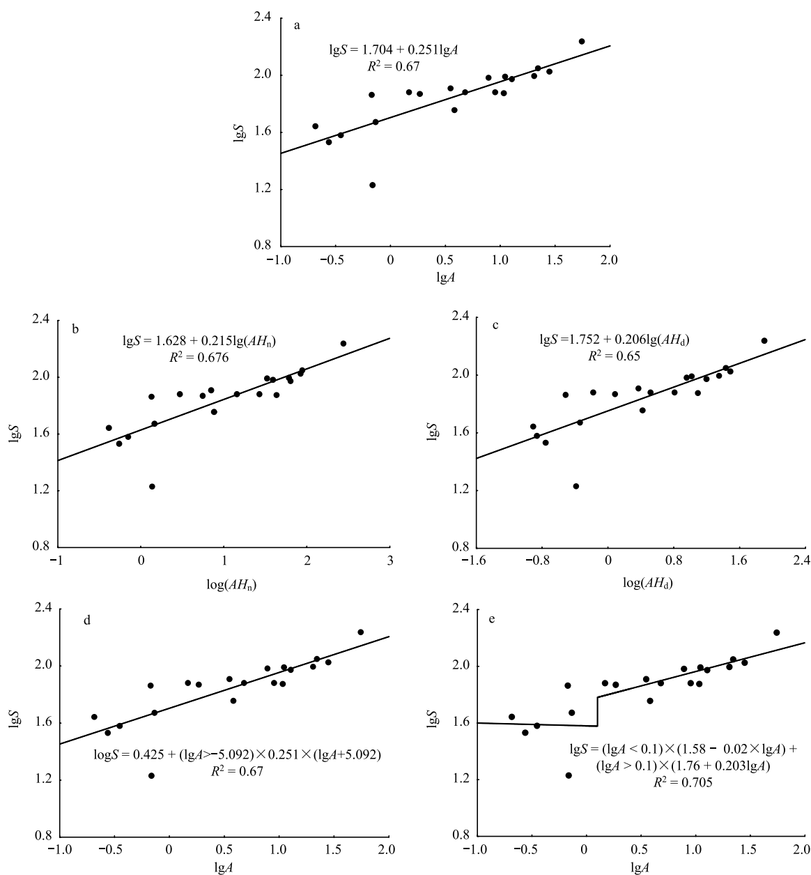
图2 基于20个小型岛屿植物丰富度拟合的种—面积关系模型
