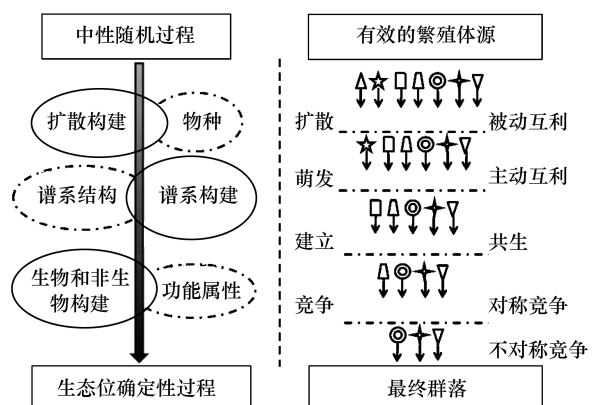
图1 中性随机和生态位过程在群落构建过程中的作用模式(图右仿自 Stokes & Archer, 2010)
