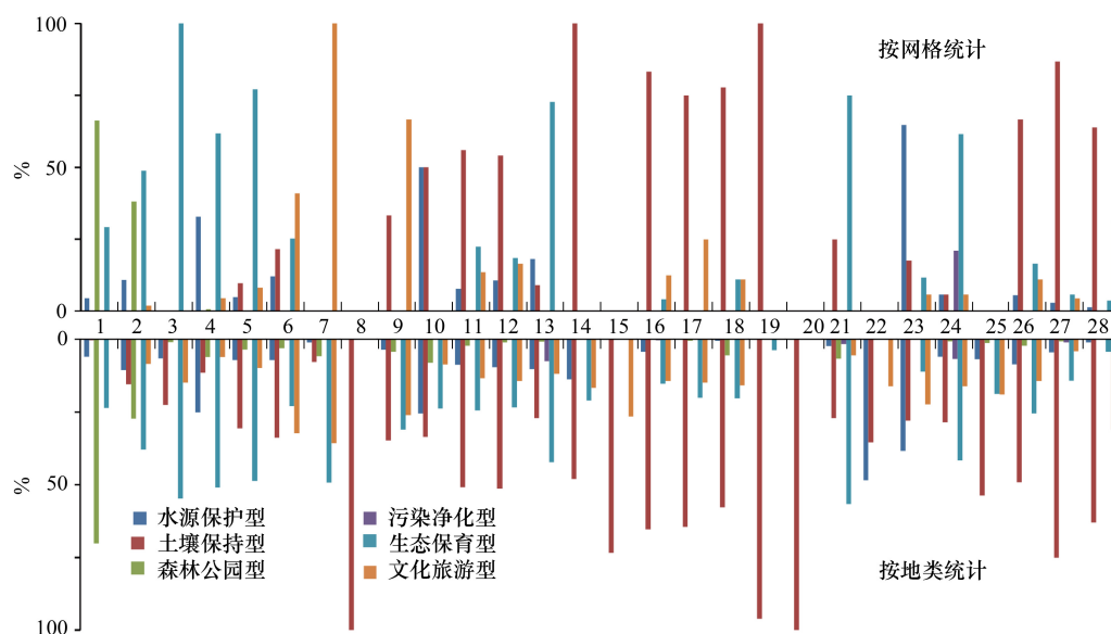
图3 土地利用类型与生态系统服务簇类型关联关系统计图
