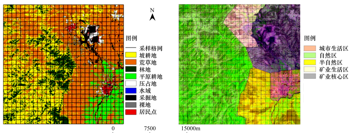
图1 研究区景观分类及功能分区
