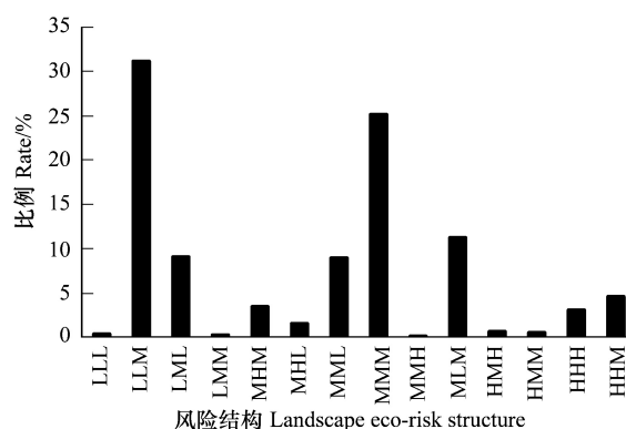
图4 矿区景观生态风险结构统计
