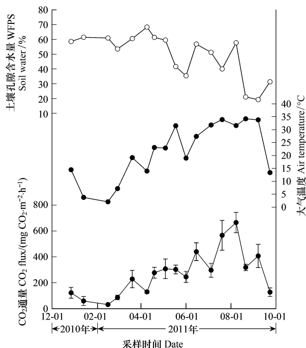
图 3 轮作期内 CO 2 通量、大气温度以及 WFPS 季节变化
