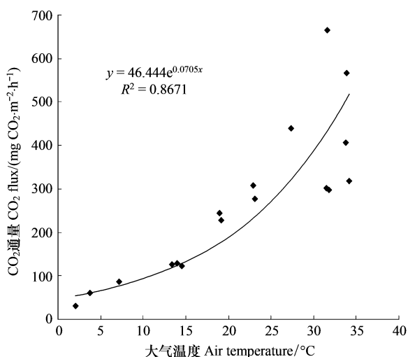
图 4 土壤 \text{CO}_2 通量与大气温度的关系
