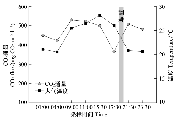
图 2 受扰动后土壤 CO 2 通量及气温昼夜变化
