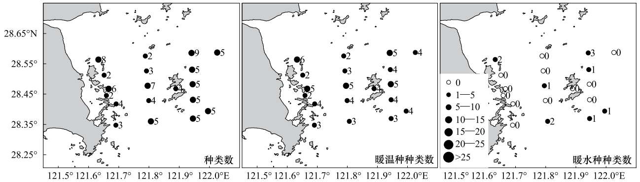
图 2 4 月浮游动物种类数分布 Fig. 2 Distribution of species richness for zooplankton in April, 2010
