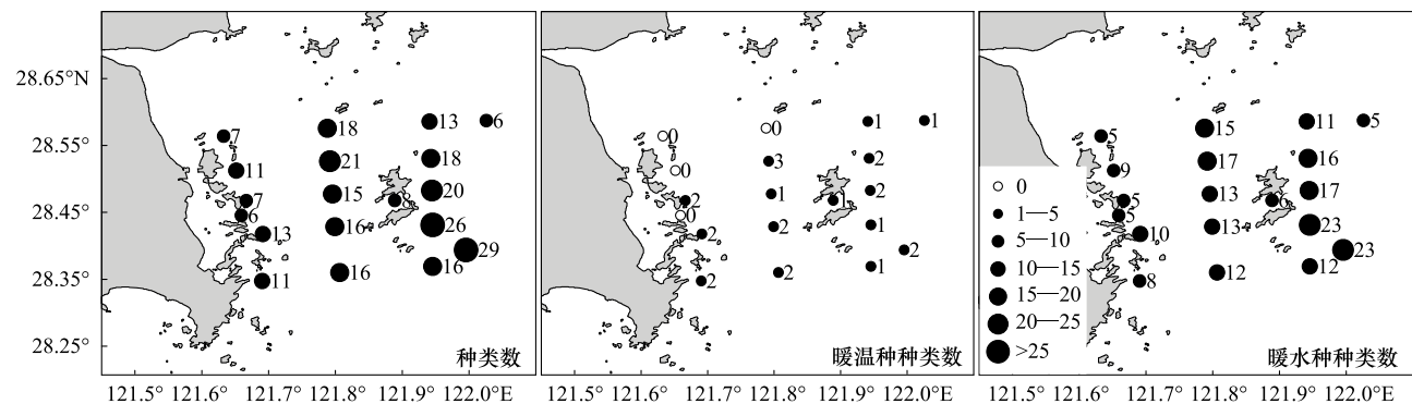
图 4 10 月浮游动物种类数分布 Fig. 4 Distribution of species richness for zooplankton in October, 2010
