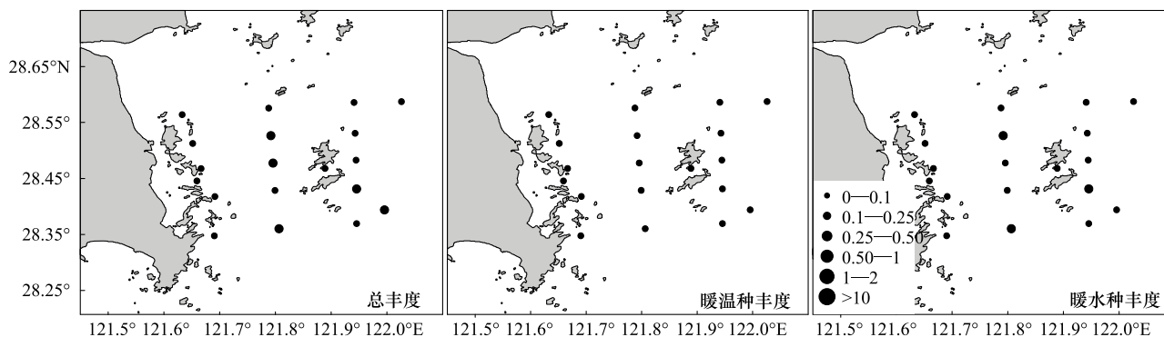
图7 调查海域10月浮游动物丰度平面分布( 10^3 个/ m^3 )
