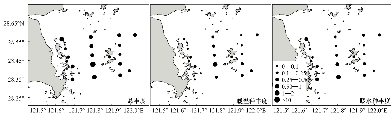
图6 调查海域7月浮游动物丰度平面分布( 10^3 个/ m^3 )
