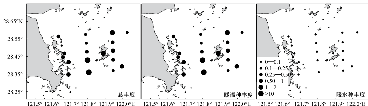
图5 4月浮游动物丰度分布( 10^3 个/ m^3 )
