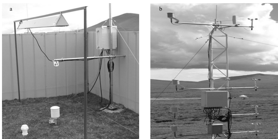
图2 增温样地 (a) 与小型生态气象观测站 (b)
