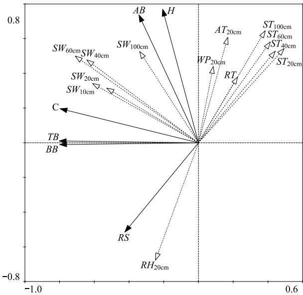
图 5 植被特征(实线)与温度、水分因子(虚线)的 RDA 排序图
